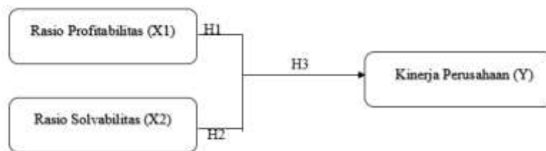
Gambar 1 Kerangka Konseptual
